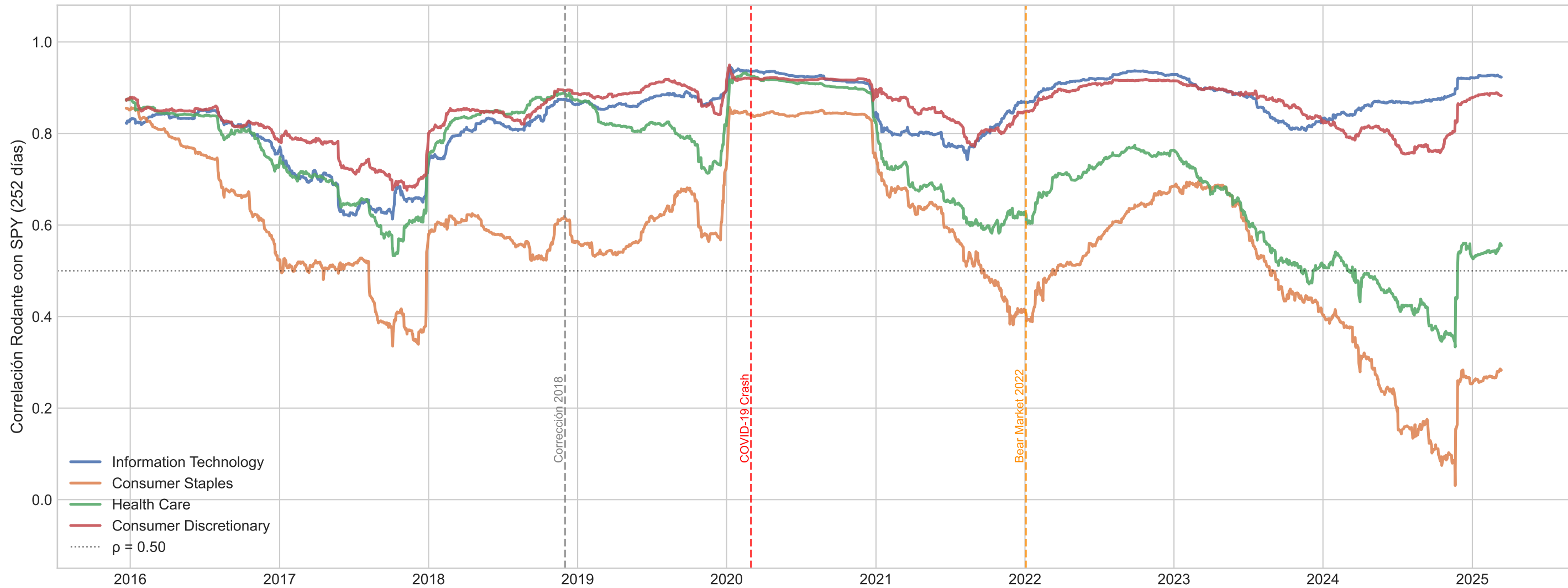
Correlación Rodante de Sectores GICS vs Benchmark — Ciclos de Mercado
