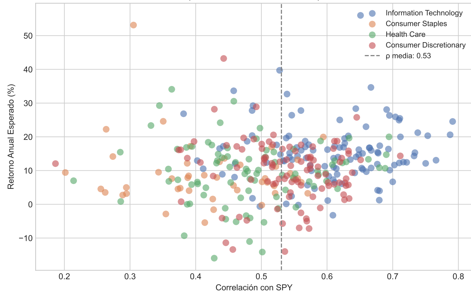
Correlación vs Retorno Anual (identificar diversificadores)
