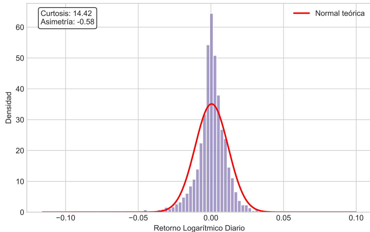
Distribución de Retornos Diarios — SPY
