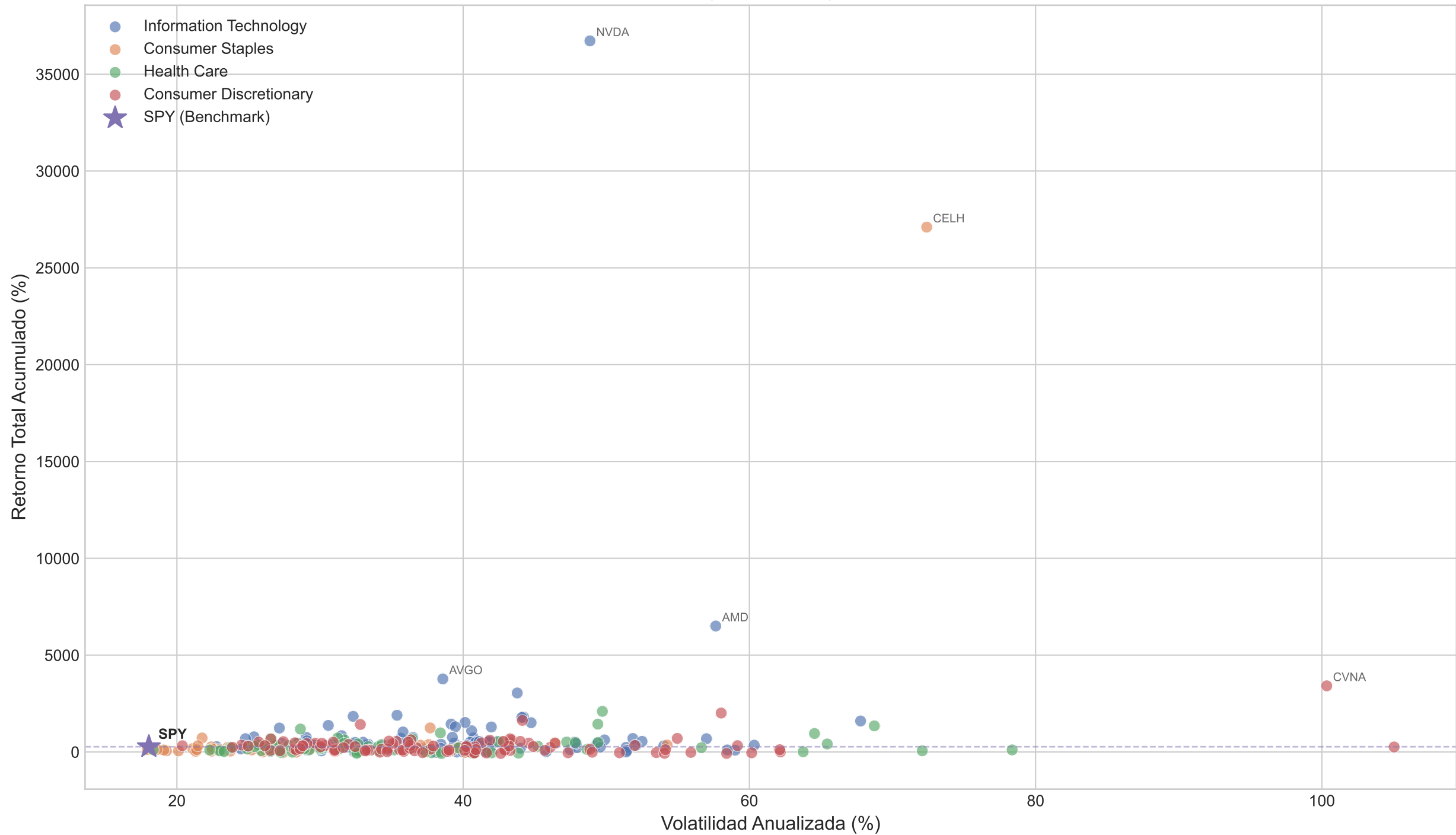
Retorno Total vs Volatilidad por Activo y Sector GICS (2015 – 2025)
