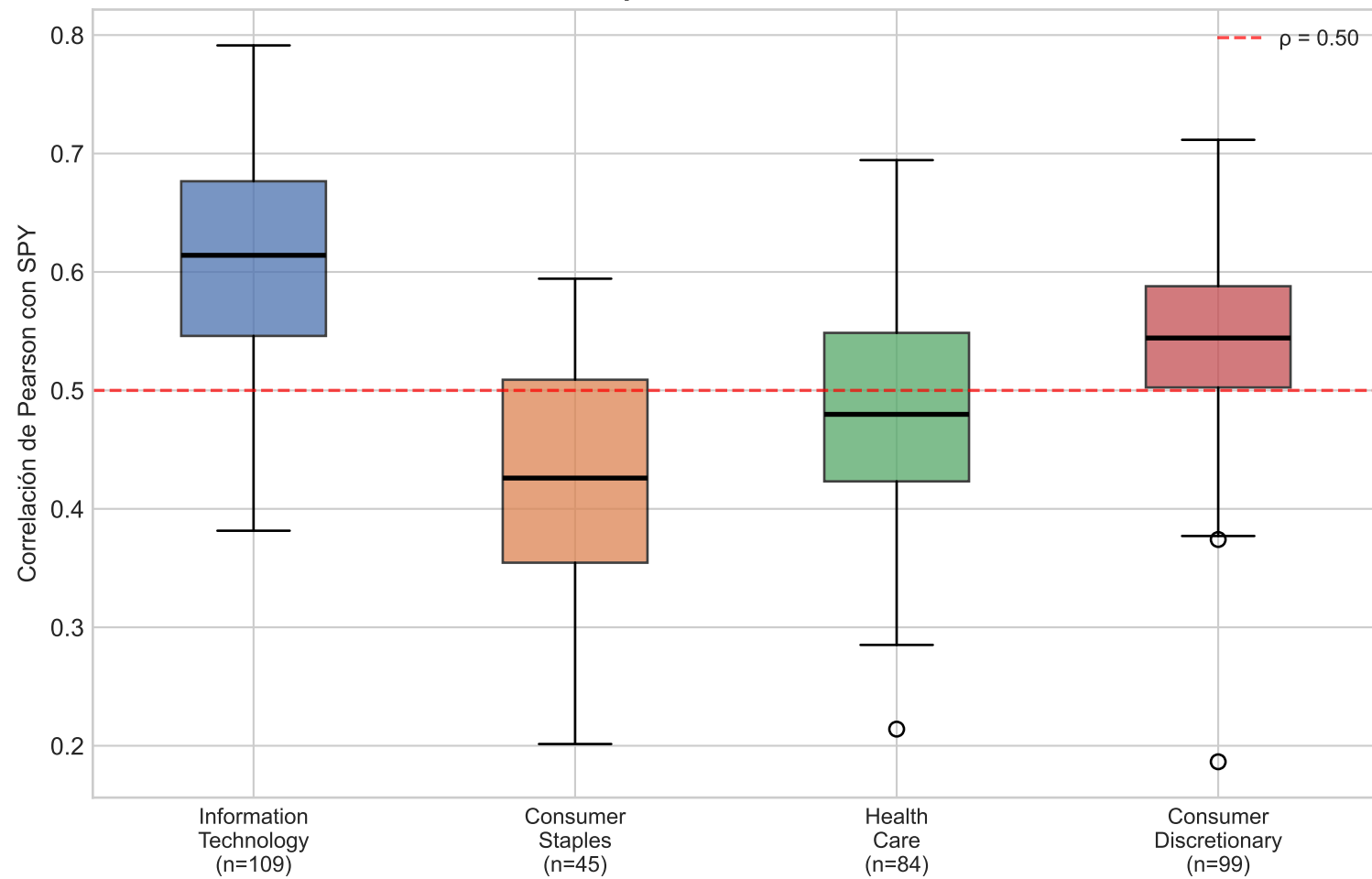
Correlación con Benchmark SPY por Sector GICS
