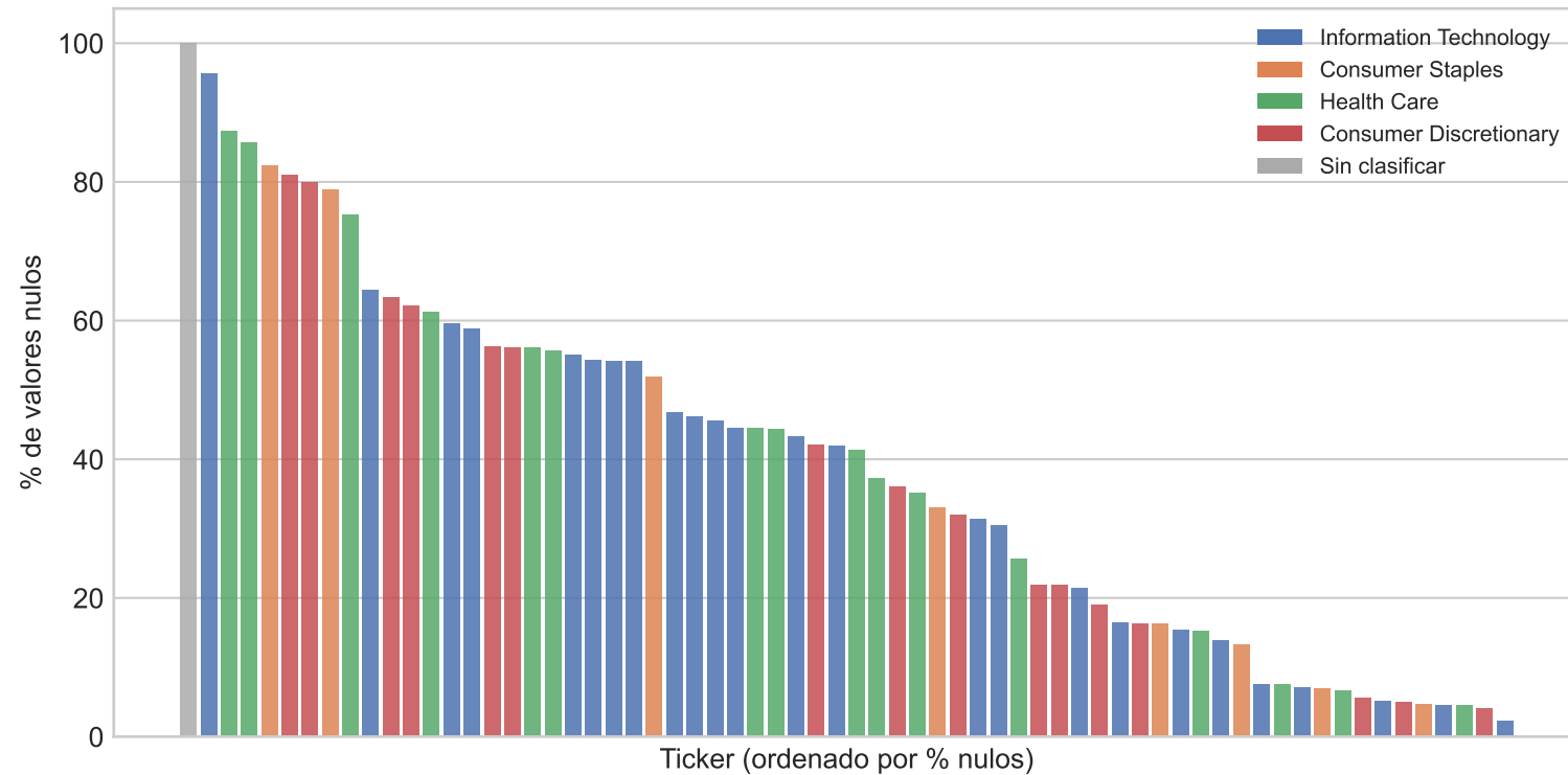
Activos con valores faltantes (coloreados por sector GICS)
