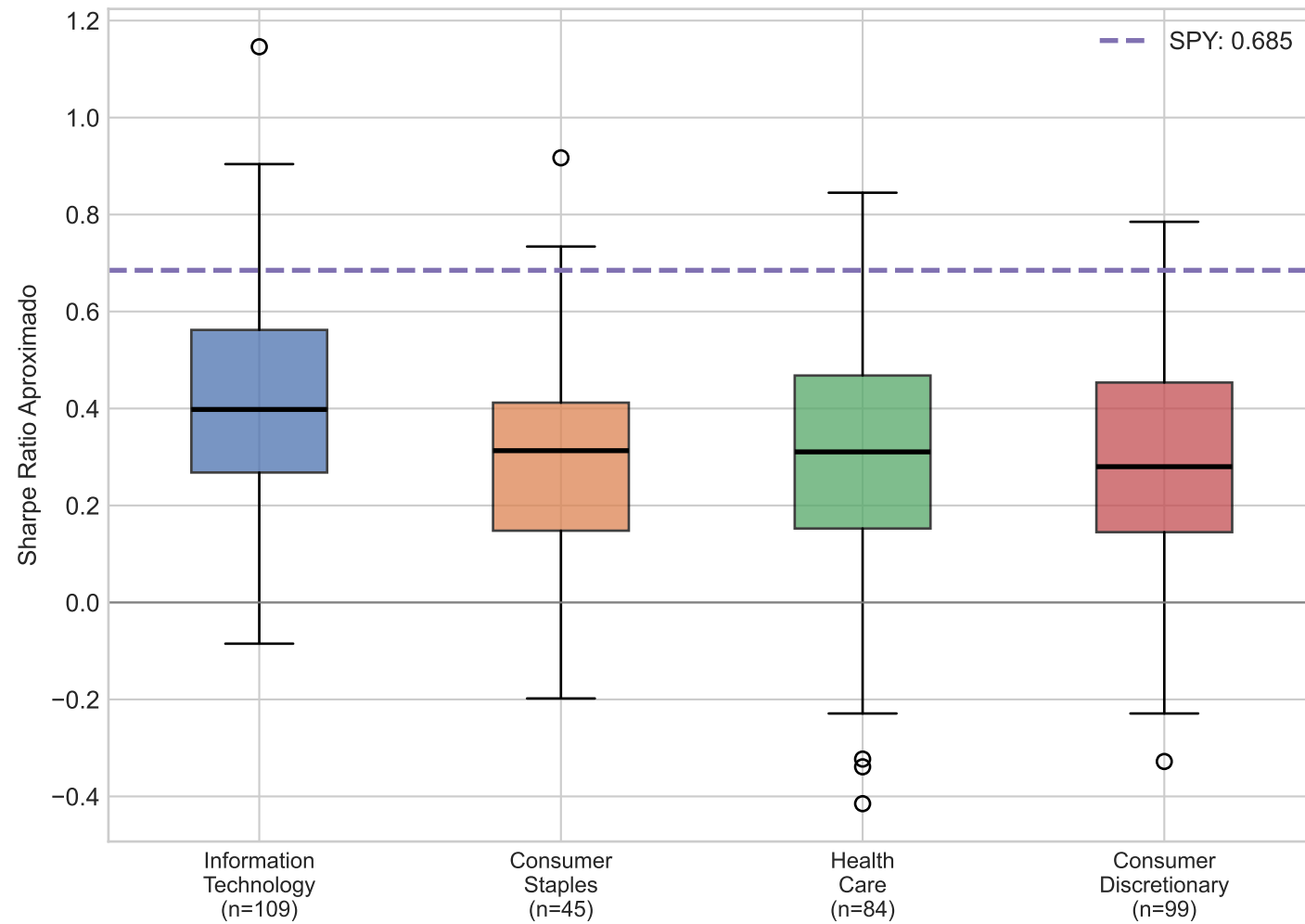
Sharpe Ratio por Sector vs Benchmark
