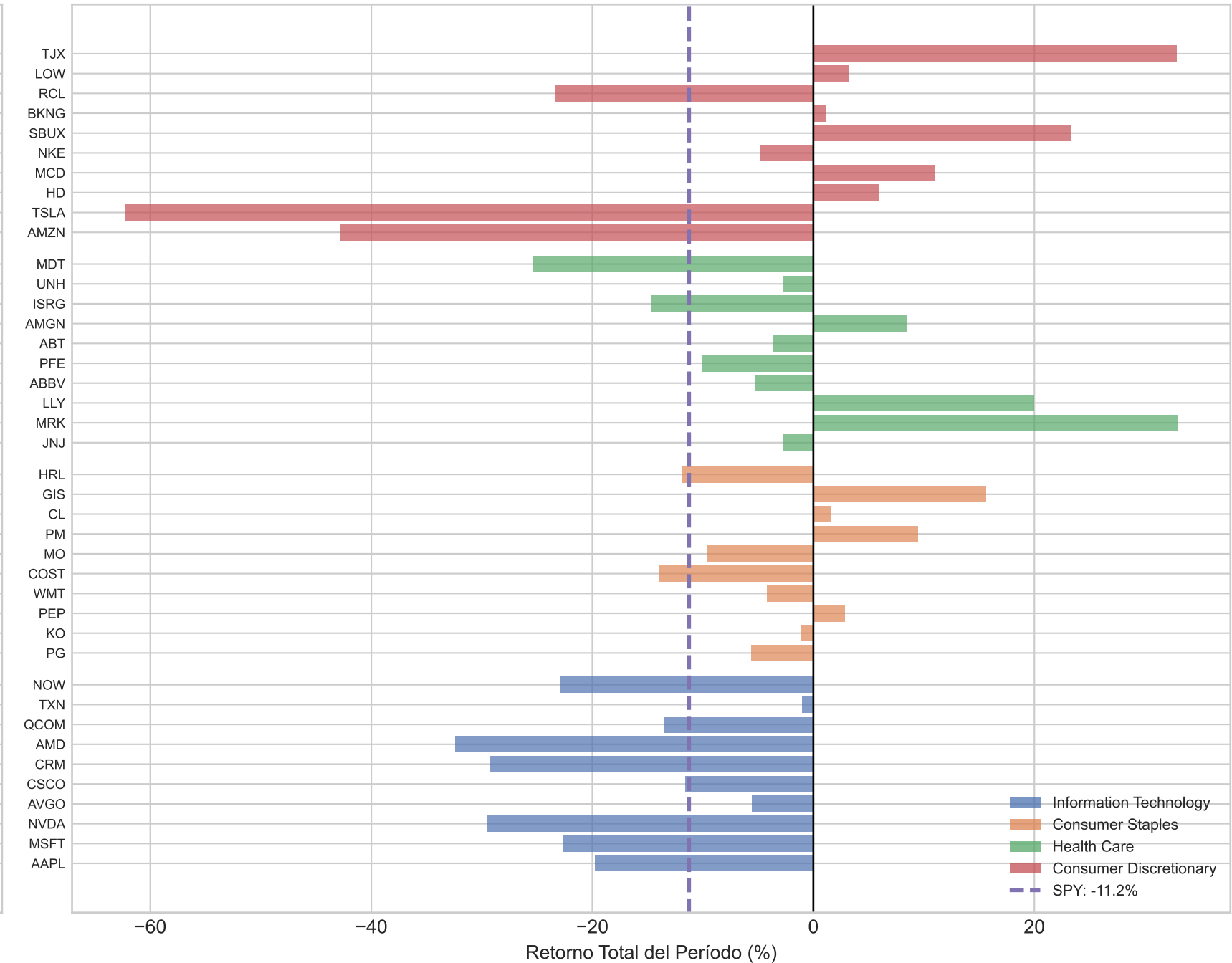
Bear Market 2022 (3 ene – 12 oct 2022)
