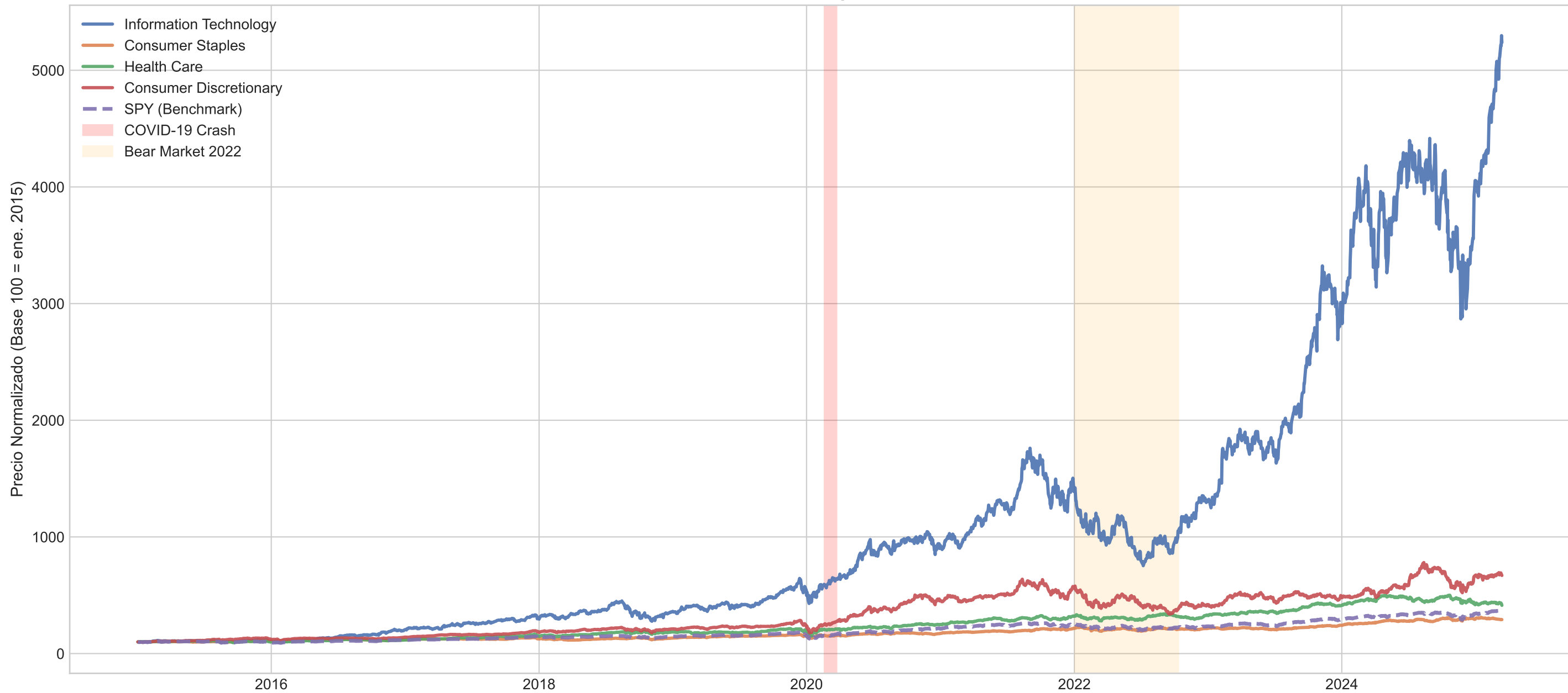
Evolución del Precio Normalizado por Sector GICS — 2015–2025
