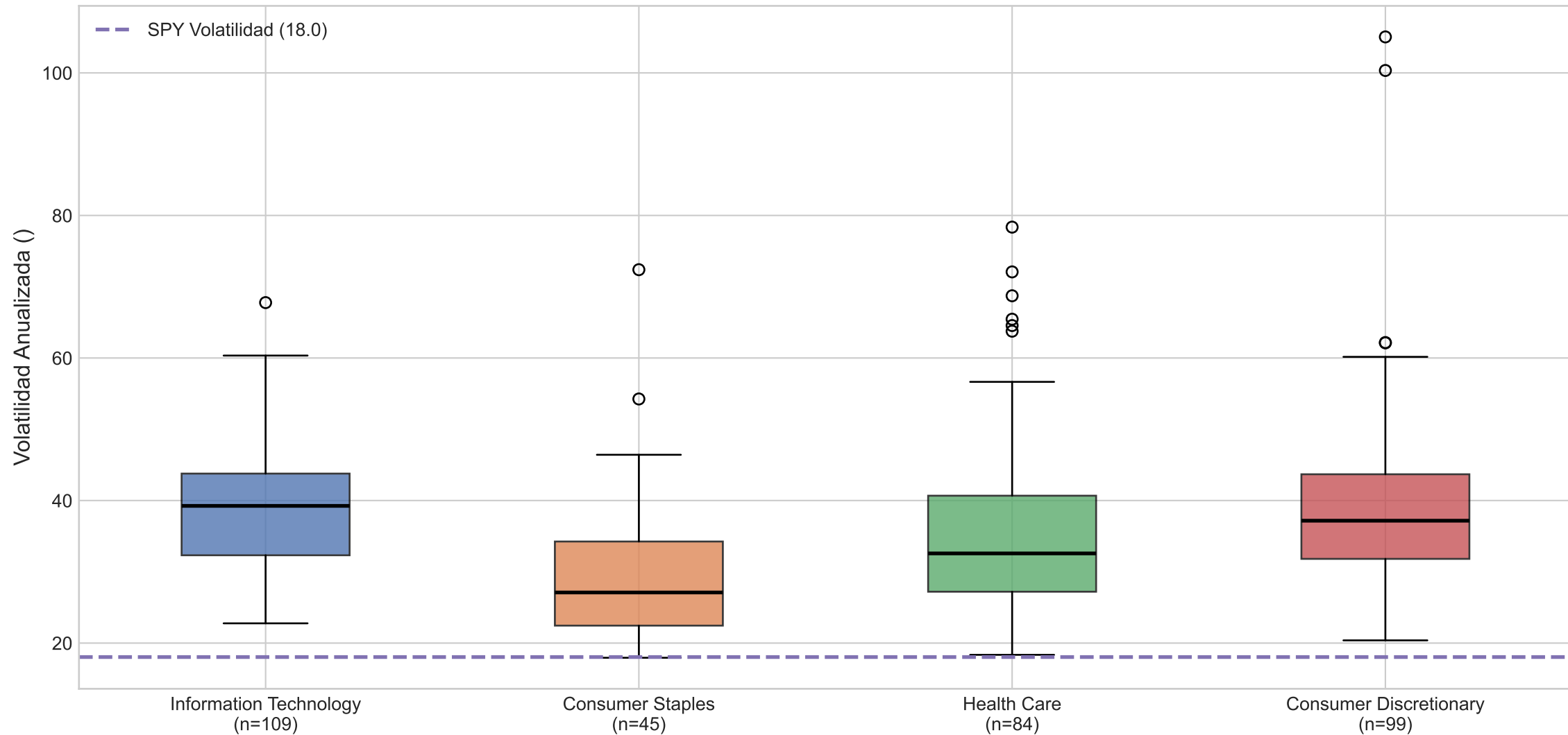
Comparativa de Volatilidad por Sector GICS vs Benchmark
