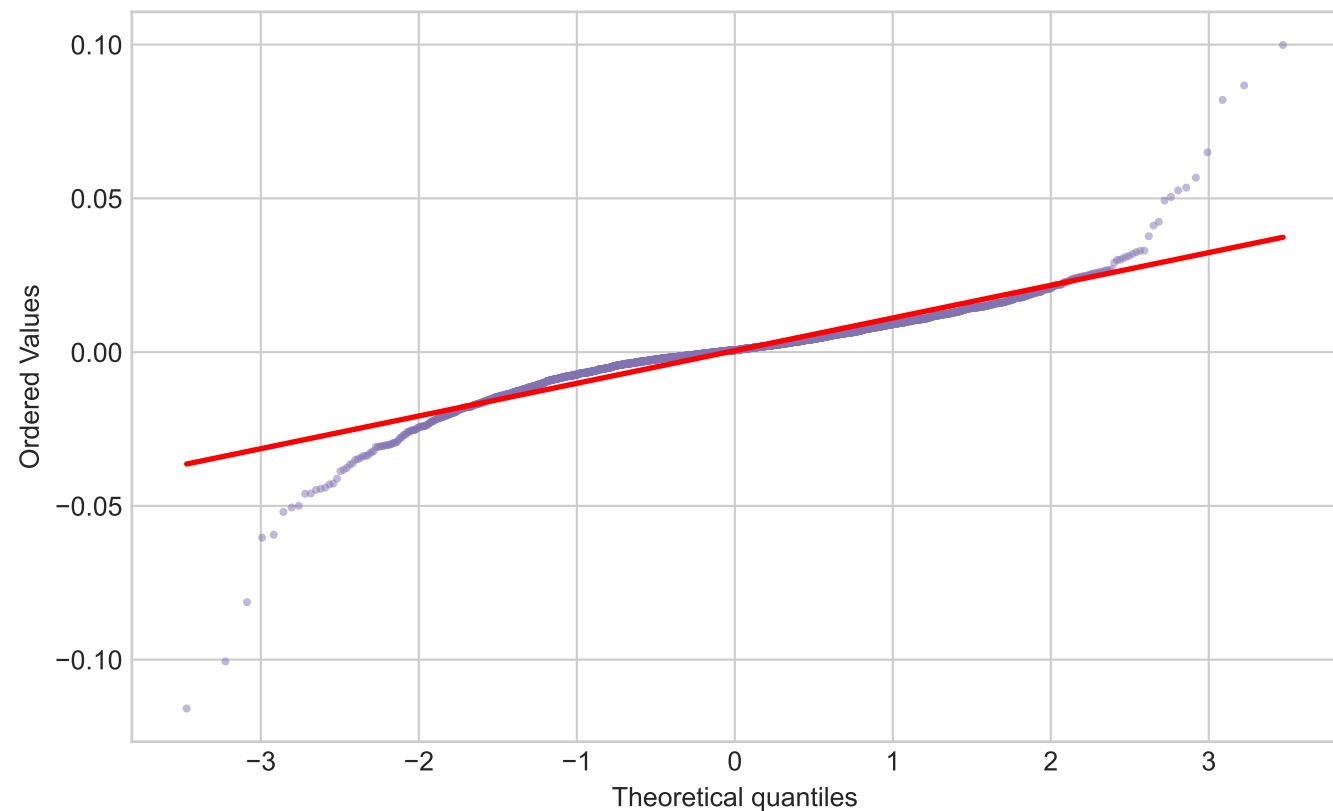
Q-Q Plot — SPY vs Distribución Normal
